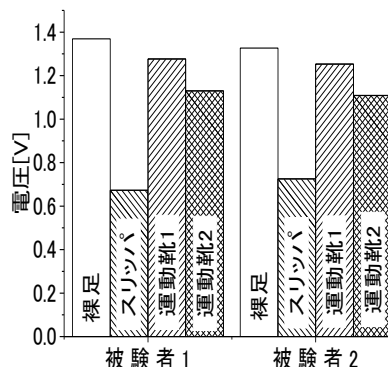
図1 靴の種類を変えた時の電圧値比較
